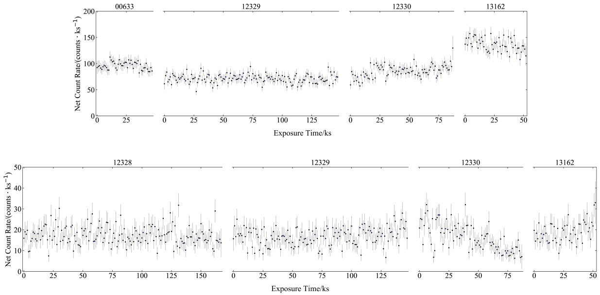
图 3 MTT68的X射线光变曲线(上)及MTT71的X射线光变曲线(下). 光变曲线上的“12329”等数字标号为相应的观测编号. 单次观测内每个数据点间隔为1 ks, 误差棒表示标准差的大小( 1\sigma ).
