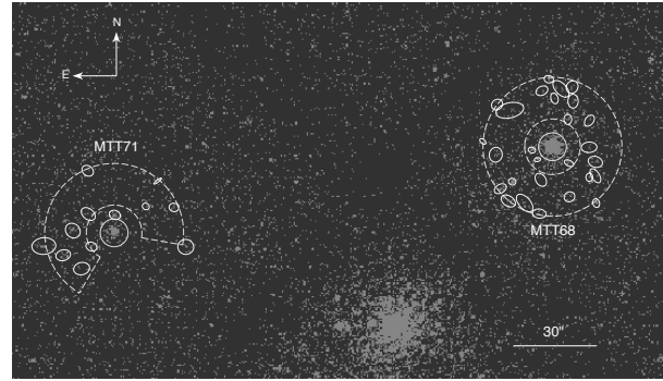
图 2 Chandra /ACIS-I在0.5–8.0 keV能段光子计数图, 其中圆圈与扇形区域为选取的MTT68和MTT71的源和背景区域, 椭圆表示探测到的需要扣除的点源.
