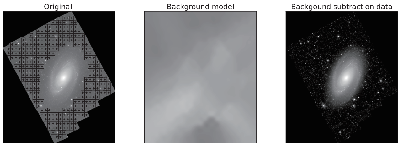
图3 M81在Spitzer-IRAC 4.5 \mu\text{m} 波段的观测图像(左图)、背景模型图像(中图)、扣除背景之后的图像(右图). 左图中黑色方框表示用于背景模型建模所用到的局部背景的区域, 黑色区域是没有观测的区域. 为了清楚显示背景的空间变化, 我们增强了背景图像的对比度.
